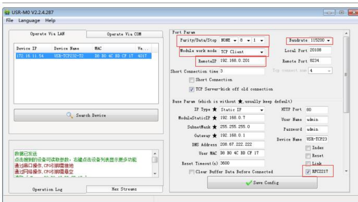
Diagram 5.1.1-4 Serial parameters
